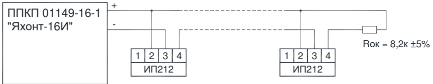
Тип ШС "АКТИВ"
