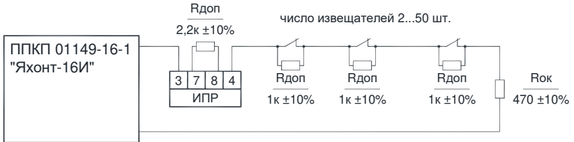
Тип ШС "ПАССИВ С ВНИМАНИЕМ"
