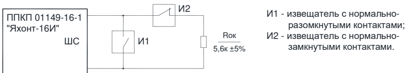
Только для ШС типа "ОХРАННЫЙ"
